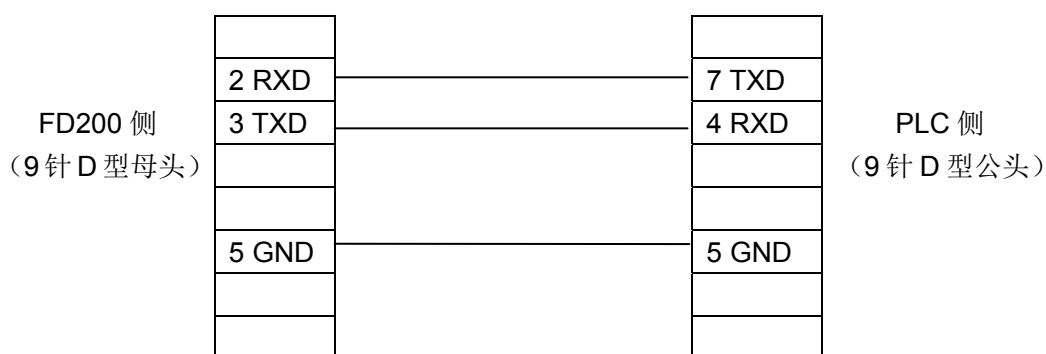
通讯电缆连线图
