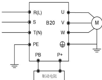
图 1-4 变频器与制动组件接线图
