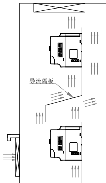
图 2-2 多台变频器的安装示意图
