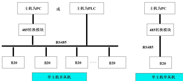
图 2-9 通讯端子配线图
