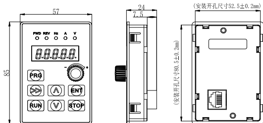
图 1-1 远控键盘 1 (B20-LKD)
