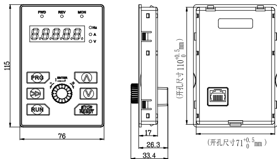
图 1-2 远控键盘 2 (B25-LKD)
