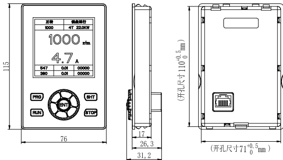
图 1-3 远控键盘 3 (B25 液晶键盘-LKD)
